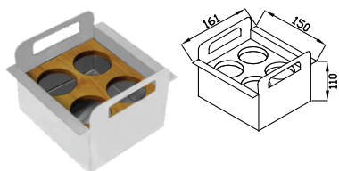
PORTA CONDIMENTOS 150 NÃO ACOMPANHA FRASCOS REF. 20.04.00144 • 150mm
